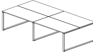
ILHA 4 POSTOS (P/ PAINEL VIDRO) 2800 X 1600 X 740 | 3600 X 1600 X 740 3200 X 1600 X 740
