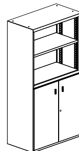
ARMÁRIO MISTO PORTAS MELAMINA/MADEIRA 1530 X 800 X 450 | 1950 X 800 X 440
