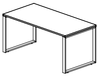
SECRETÁRIA 800 X 650 X 740 | 800 X 800 X 740 1200 X 650 X 740 | 1200 X 800 X 740 1400 X 650 X 740 | 1400 X 800 X 740 1600 X 650 X 740 | 1600 X 800 X 740 1800 X 650 X 740 | 1800 X 800 X 740
