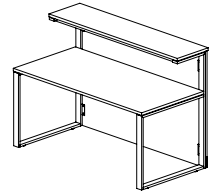
BALCÃO 800 X 800 X 1135 | 1600 X 800 X 1135 1200 X 800 X 1135 | 1800 X 800 X 1135 1400 X 800 X 1135
