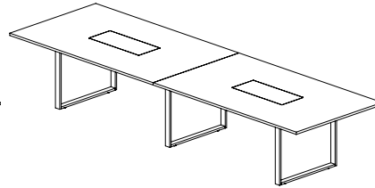
MESA REUNIÃO C/ VIDRO 4000 X 1200 X 740
