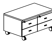
BLOCO RODADO - FRENTE MELAMINA/MADEIRA 465 X 880 X 530
