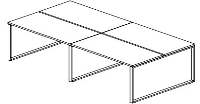
ILHA 4 POSTOS (P/ PAINEL MELAMINA) 2800 X 1600 X 740 | 3600 X 1600 X 740 3200 X 1600 X 740
